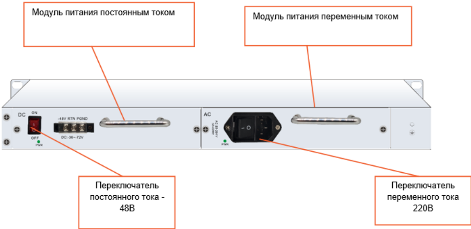
Рис.4.2 Задняя панель FG-FOM-MS-4-OTN
